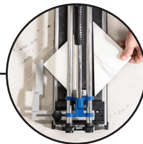
45° Angle Cuts
