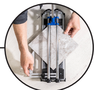
45° Angle Cuts
